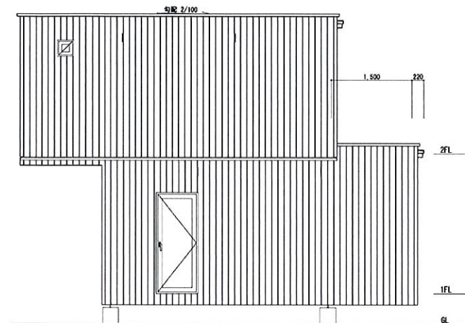
【立面図】
